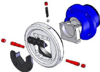
PALIER A PIECES D'USURE Detail axes d'articulation et verrouillage du volant MBC Guttin
