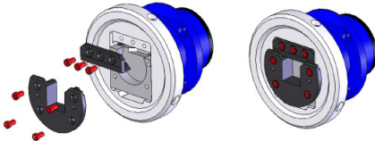
PALIER A PIECES D'USURE Montage des pieces d'usure par la face avant avec feuille d'entraînement sur le volant MBC Guttin
