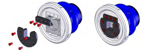
PALIER A PIECES D'USURE Montage des pièces d'usure par la face avant avec feuille d'entraînement sur le volant
