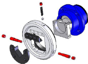
PALIER A PIECES D'USURE Detail axes d'articulation et verrouillage du volant
