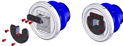
PALIER A PIECES D'USURE Montage des pièces d'usure par la face avant avec feuille d'entraînement sur le volant
